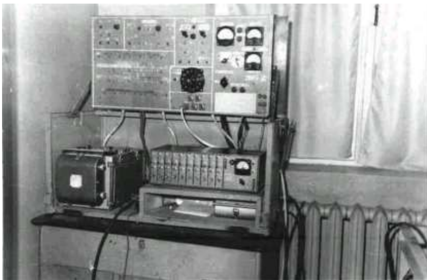
Рис. 1. Тензометрическая аппаратура.
