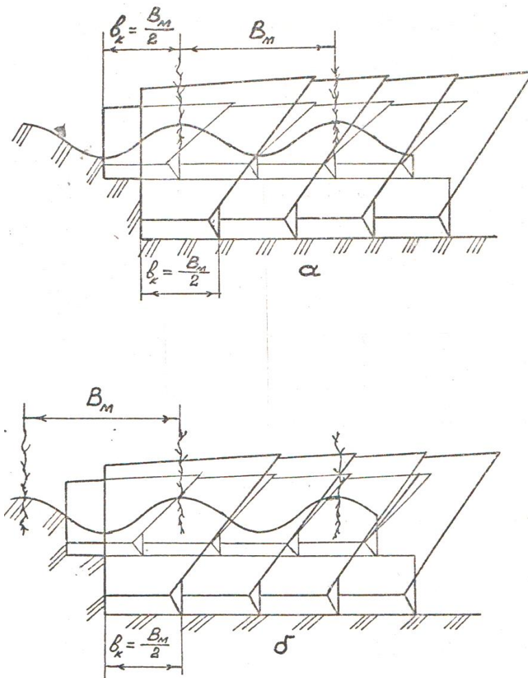
Рис. 1. Технологическая схема двухъярусной вспашки хлопковых полей
